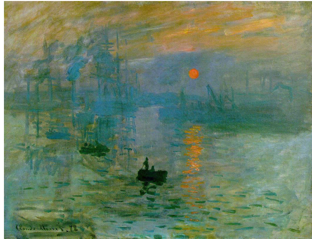
Fig. 2, Nascer do Sol, 1872
